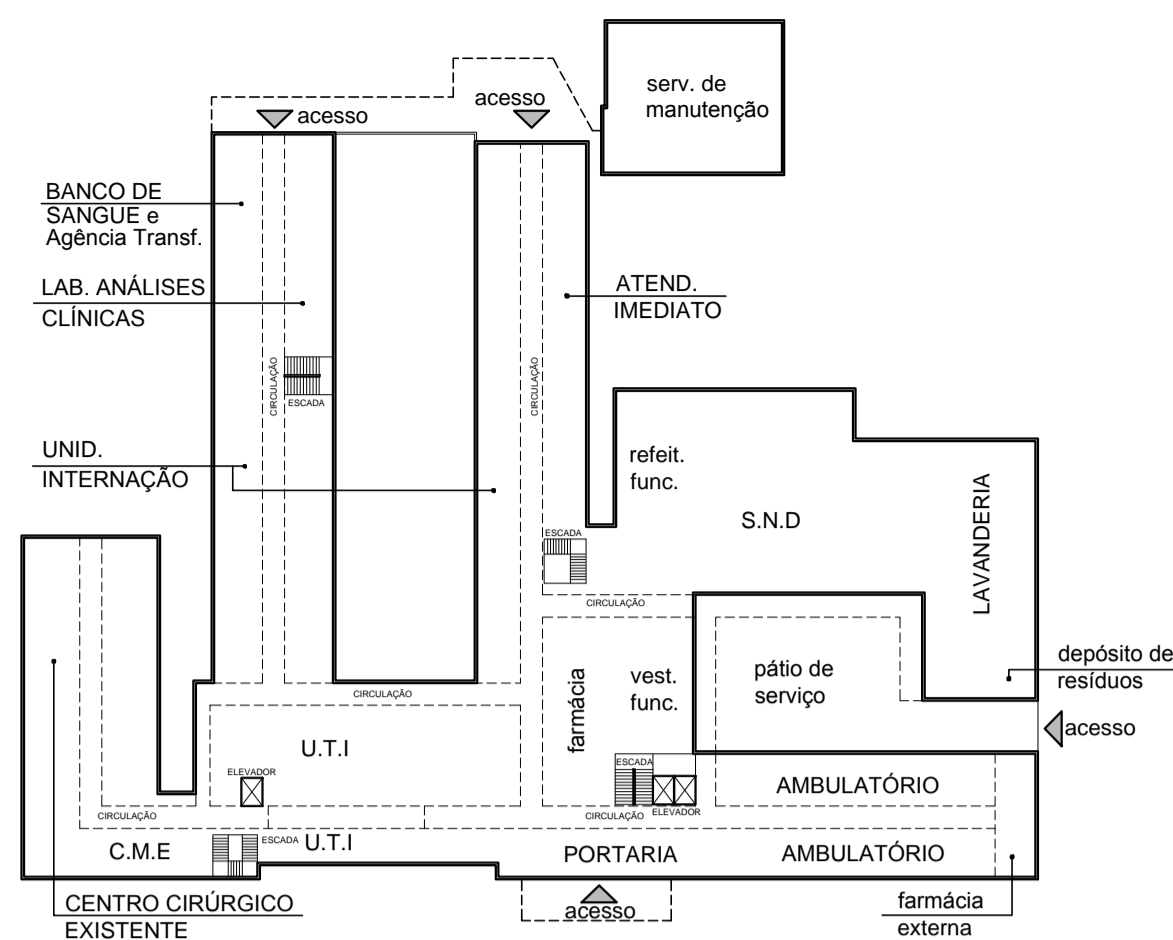
PLANTA ESQUEMÁTICA PAVTO. TÉRREO Hospital Montenegro ESCALA 1/750
